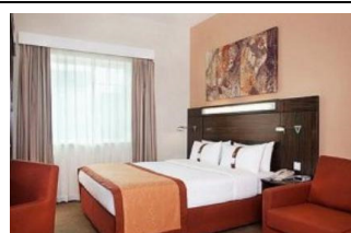
szoba példa
